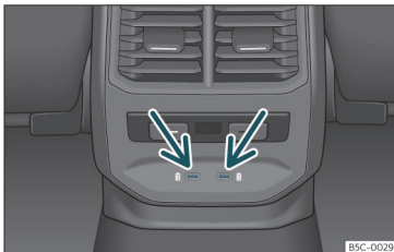
Fig. 137 Midterkonsol bag: USB-porte med stikdåsefunktion
