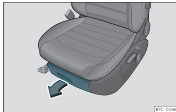
Fig. 123 | Opbevaringsrum under forsæde
