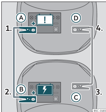
Fig. 42 Tilslutningsdiagram for biler med start-stop-system
