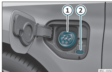
Fig. 189 Bag batteriladeklappen forrest i venstre side: ladestikdåse
