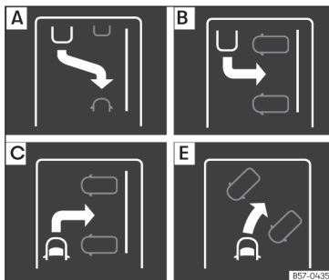
Fig. 176 På kombiinstrumentets skærm: visning af parkeringsfunktioner
