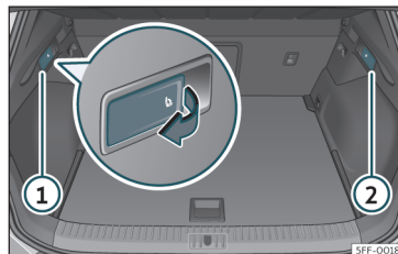
Fig. 107 I bagagerummet: greb til udløsning af bagsæderyglæn
