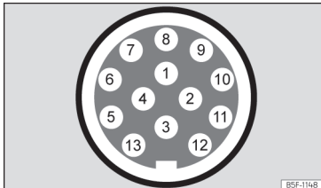
Fig. 184 Skematisk visning: tilhørsforhold for stikben i anhængerstikdåsen
