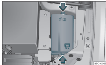
Fig. 48 I motorrummet: afdækning på sikringsboks
