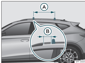
Fig. 121 Fastgørelsespunkter til længdevangerne til tagbøjlesystemet
