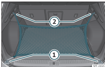
Fig. 117 I bagagerummet: øjer (1) og kroge (2) til fastgørelse af bagagenet
