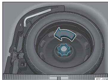
Fig. 216 | bagagerummet: bundplade, der er klappet op
