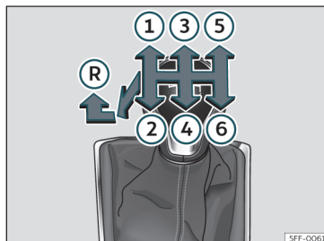
Fig. 141 Skiftediagram til 6-trins manuel gearkasse
