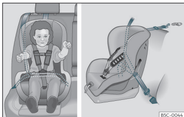
Fig. 31 På bagsædet: montering af børnesæde
