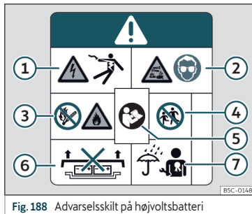
Fig. 188 Advarselsskilte på højvoltsbatteri
