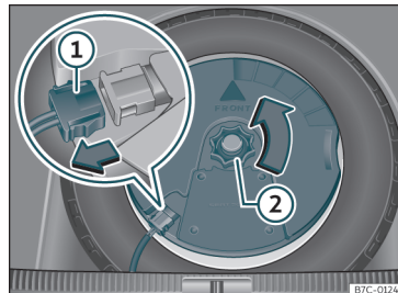
Fig. 217 | bagagerummet: afmontering af subwoofer
