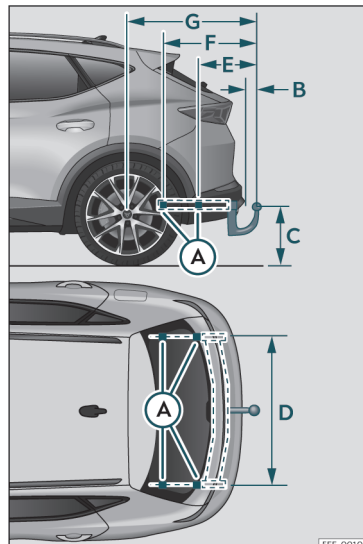
Fig. 186 Mål og fastgørelsespunkter for eftermontering af anhængertræk
