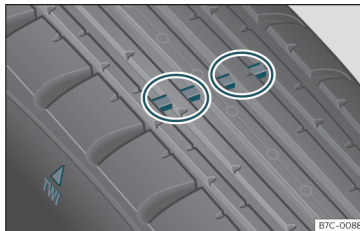
Fig. 213 Dækprofil: slidindikatorer
