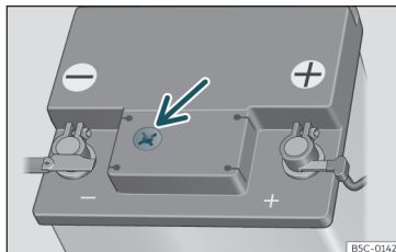
Fig. 210 Inspektionsrude på oversiden af bilens 12-volts-batteri (principskitse)
