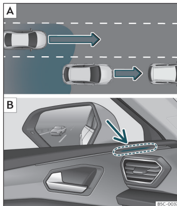
Fig. 167 Skematisk visning: A ) Overhaling med trafik i det bageste område. B ) Indikator til vognbaneskiftassistent i kontrollampe i venstre side
