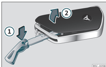
Fig. 72 Bilnøgle: åbning af afdækning til batterirum
