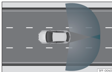
Fig. 149 Sensorernes registreringsområde
