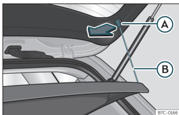
Fig. 109 I bagagerummet: af- og påmontering af bagagerumsafdækning
