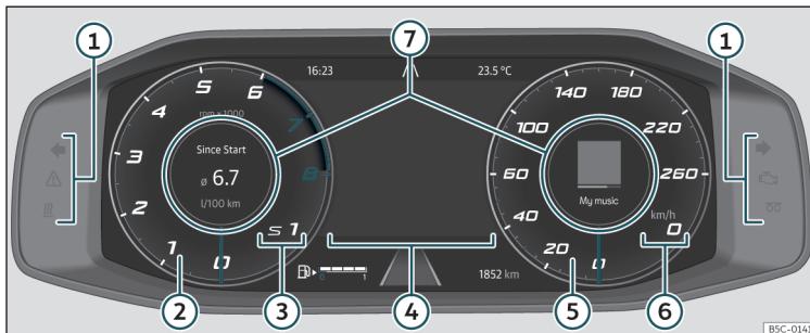
Fig. 51 Digital Cockpit i instrumentpanelet (klassisk visning)
