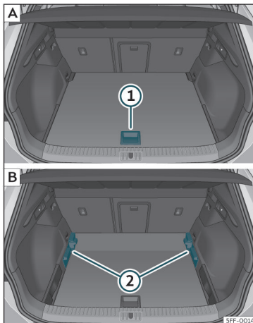
Fig. 113 Variabel bagagerumsbund: [A] høj indstilling; [B] lav indstilling
