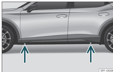
Fig. 38 Løftepunkter til donkraften
