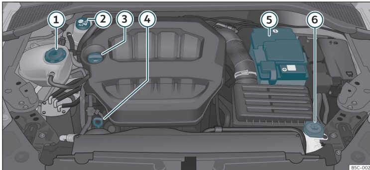
Fig. 202 Elementernes placering
